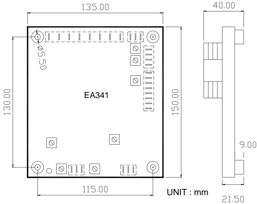
图一 外型尺寸图
