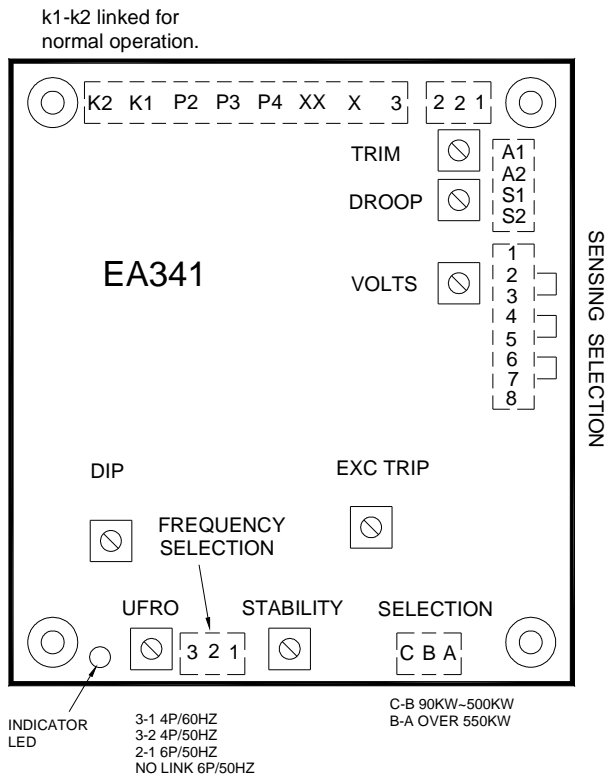
图二 外型配置图
